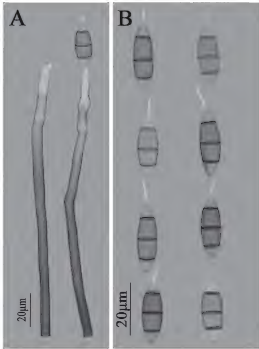
FIG. 2. Endophragmiella pulchra .
